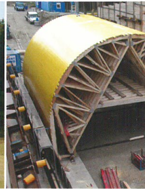
Grünbrücke - November 2016 Schalungswagen
