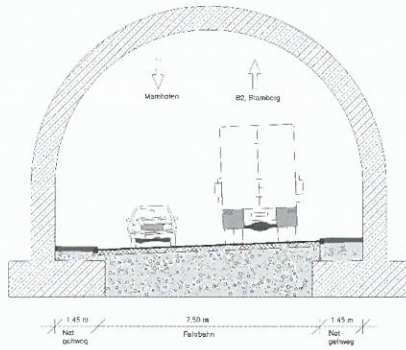
Grünbrücke - Querschnitt Fahrbahnbreite: 7,5 m
